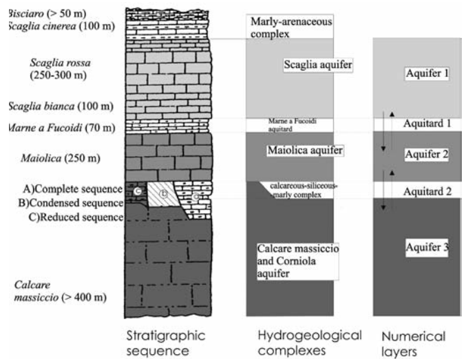
Fig. 3 - Schematizzazione dei rapporti fra successione stratigrafica umbromarchigiana, complessi idrogeologici (acquiferi, aquitards e aquicludes) in cui sono raggruppate le litologie e strati per il modello numerico (da PREZIOSI, 2007) - Schematic representation of the relations among the stratigraphic succession of the Umbria-Marche area, the hydrogeological complexes (aquifers, aquitards and aquicludes) into which the lithologies are grouped and the layers of the numerical model (from PREZIOSI, 2007)
