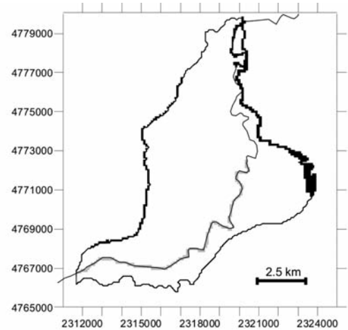
Fig. 11 - Condizioni al contorno del modello. Celle nere: flusso costante (106 l/s ai confini esterni e 180 l/s lungo il Chiascio); celle grigie: condizioni di dreno; celle bianche all'interno del dominio: ricarica da infiltrazione efficace. Dove non specificato diversamente sui confini esterni del dominio è stata assegnata una condizione di flusso nullo - Model boundary conditions. Black cells: constant flow (106 l/s at the external boundaries and 180 l/s along Chiascio river); grey cells: drain condition; white cells inside domain: recharge by effective rainfall infiltration. Where not otherwise specified a no-flow boundary condition has been assigned on the edge of the domain
