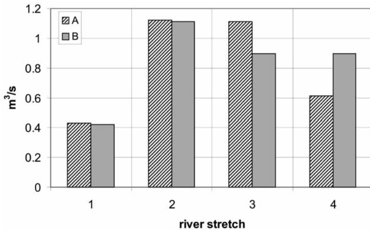
Fig. 6 - Confronto fra portata osservata (a: media aritmetica dei valori misurati nel periodo di osservazione) e la portata calcolata dal modello numerico in regime permanente (B) per ogni tratto di fiume considerato come sorgente lineare (1-4 da monte verso valle) - Comparison between observed discharge (A: arithmetic mean of the values measured during the observation period) and the discharge calculated by the steady state model (B) for each stretch of river considered as a linear spring (1-4 in a downstream direction)
