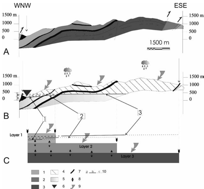
Fig. 4 - Relazioni fra (A) assetto geologico, (B) acquiferi e (C) modello numerico mostrate in un profilo schematico attraverso Monte Coscerno (modificato da Preziosi, 2007). LEGENDA: 1) acquifero della Scaglia; 2) acquifero della Maiolica; 3) acquifero del Calcere massiccio-Corniola; 4) zona insatura; 5) zona satura; 6) sorgente lineare; 7) limite a flusso nullo; 8) flusso di drainance; 9) infiltrazione efficace; 10) potenziale idraulico: a) imprigionato, b) libero, c) fittizio - Relations among (A) geological framework, (B) aquifers and (C) numerical model shown in a schematic cross section across Mt. Coscerno (modified from PREZIOSI, 2007). LEGEND: 1) Scaglia aquifer; 2) Maiolica aquifer; 3) Calcere massiccio-Corniola aquifer; 4) unsaturated zone; 5) saturated zone; 6) linear spring; 7) no flow limit; 8) leakage; 9) recharge; 10) aquifer potential: a) confined; b) phreatic; c) fictitious
