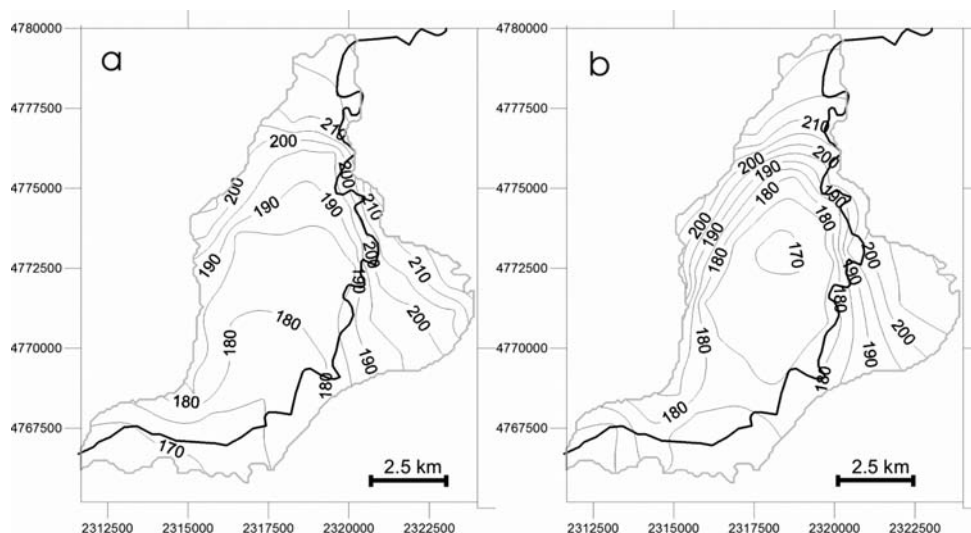
Fig. 10 - a: superficie piezometrica relativa al 1974; b: superficie piezometrica relativa al 2004 (m s.l.m.; equidistanza 5 m) - a: head contour referring to the year 1974; b: head contour referring to the year 2004 (m a.s.l.; 5 m spacing)
