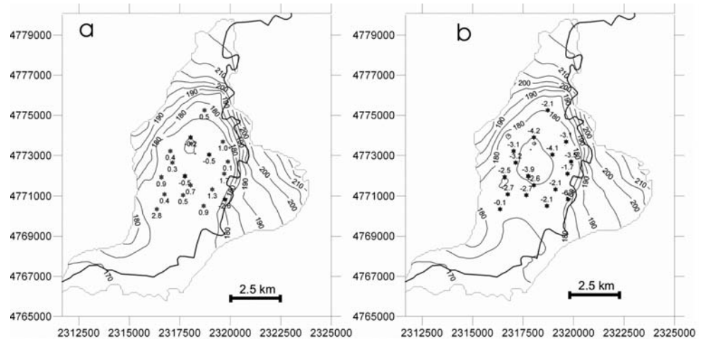
Fig. 12 - Superficie piezometrica calcolata da MOD2 (a) e MOD3 (b) in condizioni di sfruttamento dell'acquifero. I valori puntuali indicano la differenza tra l'altezza piezometrica misurata nei pozzi dell'area di studio e quella calcolata - Head contour under conditions of aquifer exploitation as calculated by MOD2 (a) and MOD3 (b). The point values indicate the difference between piezometric heads measured in the well field area and the calculated piezometric heads
